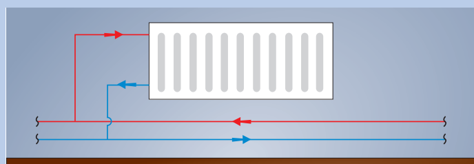
Horné a spodné pripojenie na rovnakej strane
