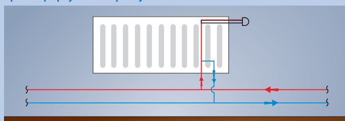
Kompaktné pripojenie ventilu (VK)
