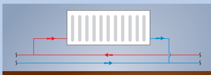
Spodné pripojenie na opačných stranách
