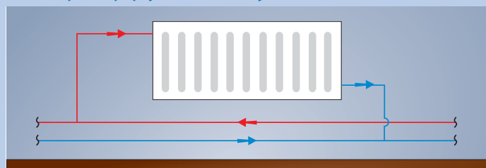
Horné a spodné pripojenie na opačných stranách
